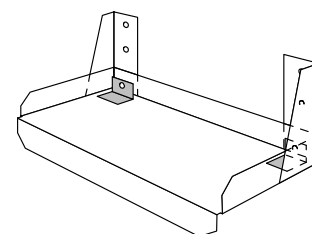
Suporte tipo Bandeja com Pontos de Fixação do Aparelho e Abas para Fixação na Parede
