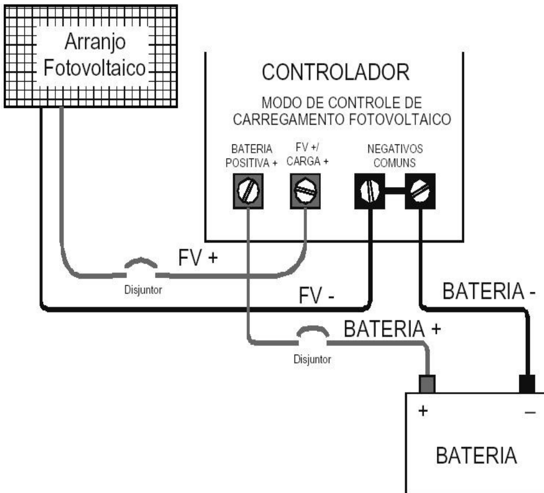
Figura 7 Diagrama de fiação de controle de carregamento fotovoltaico
